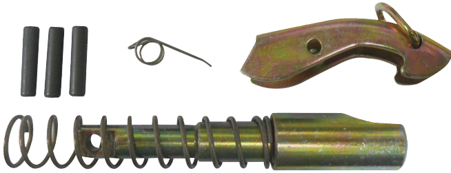
대형톱링크후크 부품
